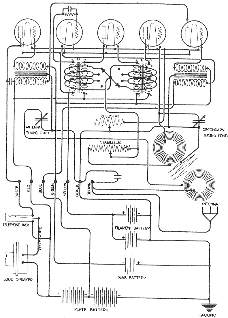
FIG. 4—SCHEMATIC WIRING DIAGRAM RADIOLA VII-B
